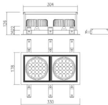
Technische Zeichnung
